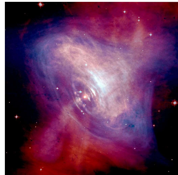
かにパルサー (かに座星雲の中心にいる中性子星)
